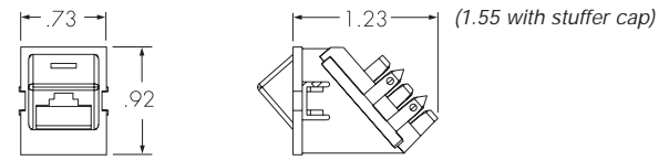
Clarity6 TracJack angled
