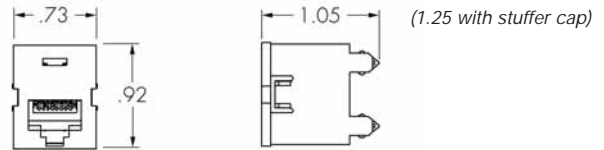
Clarity6 TracJack 180° flush
