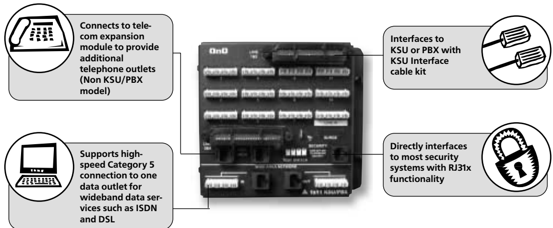
1x11 KSU/PBX Telecom Module
